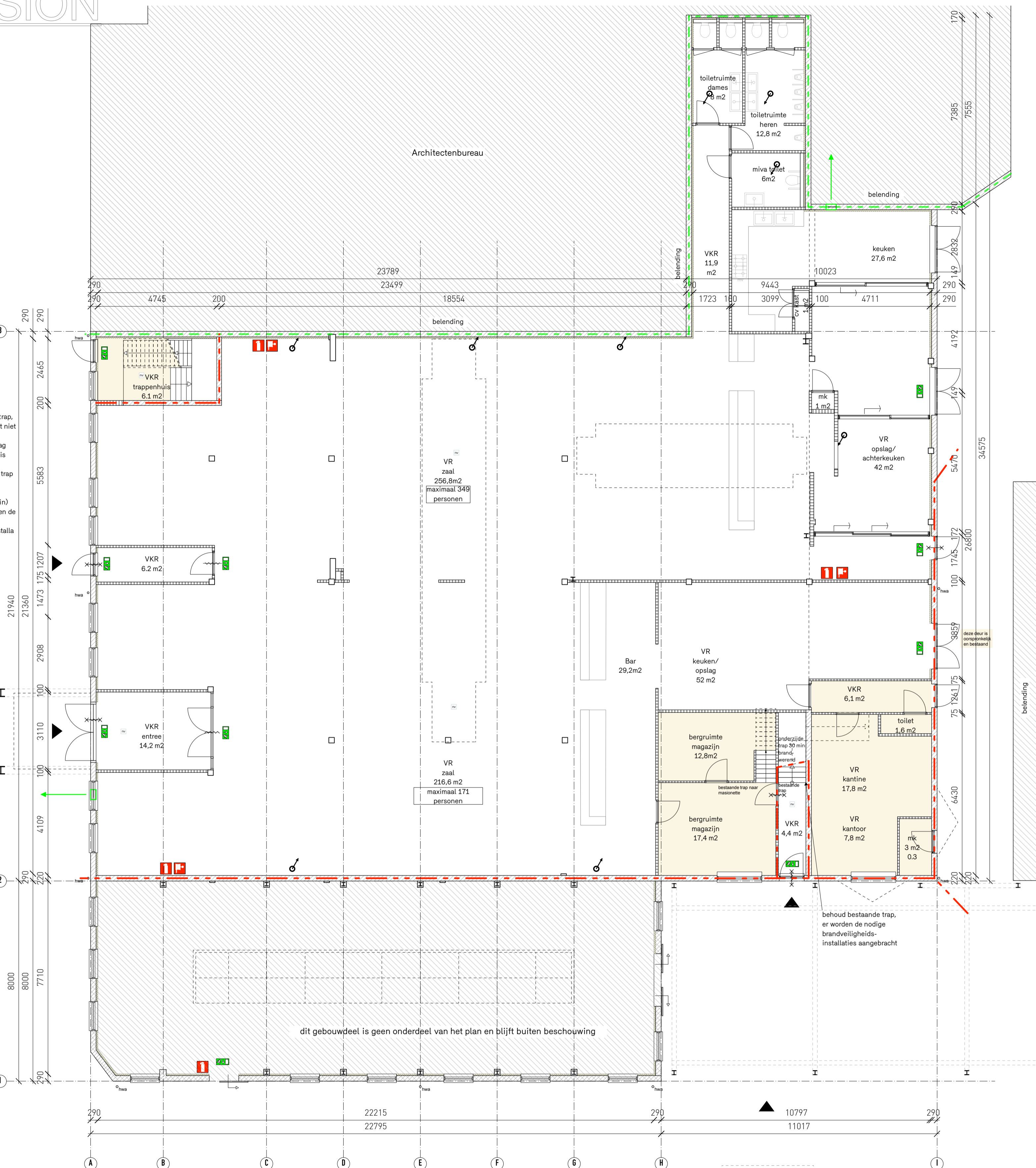
Plattegrond begane grond (nieuw-tijdelijk) 1:100
